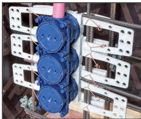
Mehrfachkombination im 71 mm Normabstand durch integrierte Kombinocken passgenau montieren.
